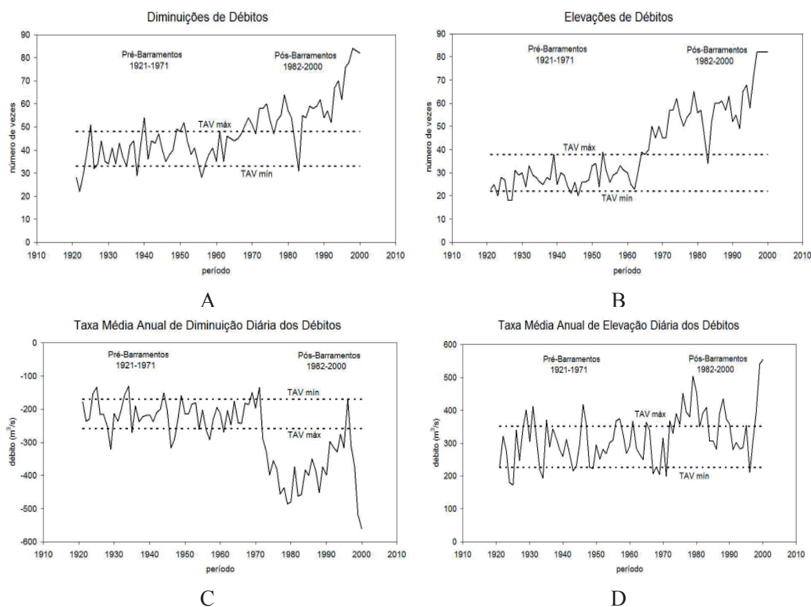
FIGURA 9: Taxa de alteração do fluxo. A e B: frequência de ocorrências de quedas e elevações nos débitos; C e D: magnitude das ocorrências de quedas e elevações no fluxo.
