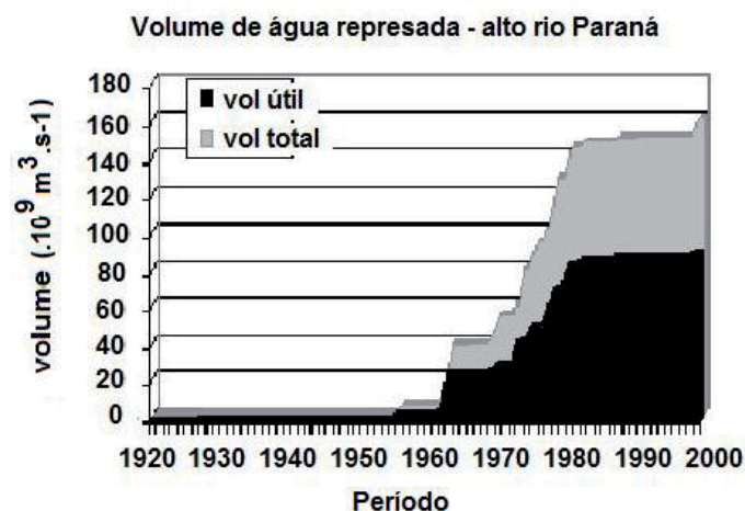
FIGURA 5. Volume total e útil de 27 grandes (maiores) reservatórios na bacia do Alto Rio Paraná.
