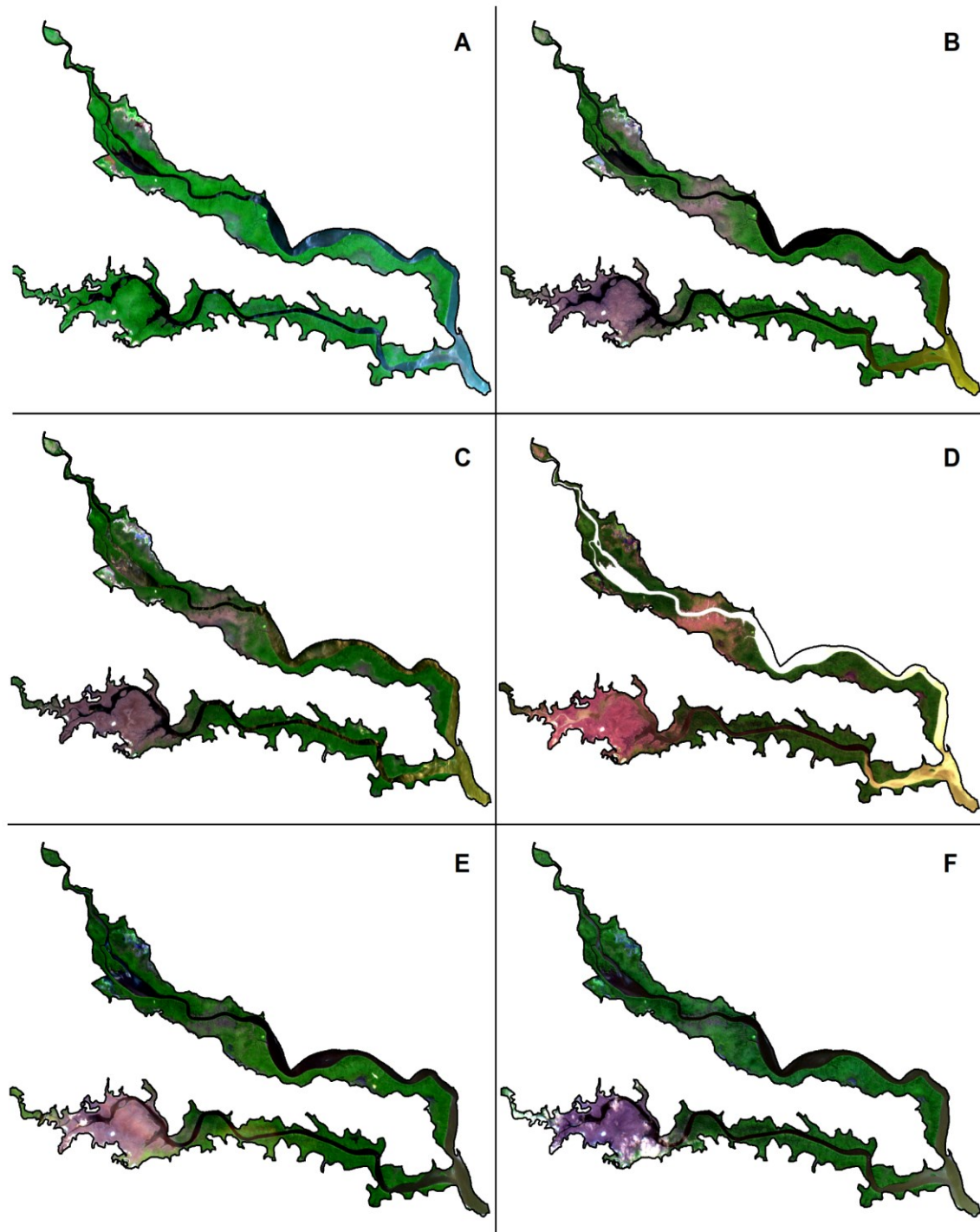
Figure 03 - Composition RGB of the Reserva de Desenvolvimento Sustentável Piraquê Açú-Mirim.
