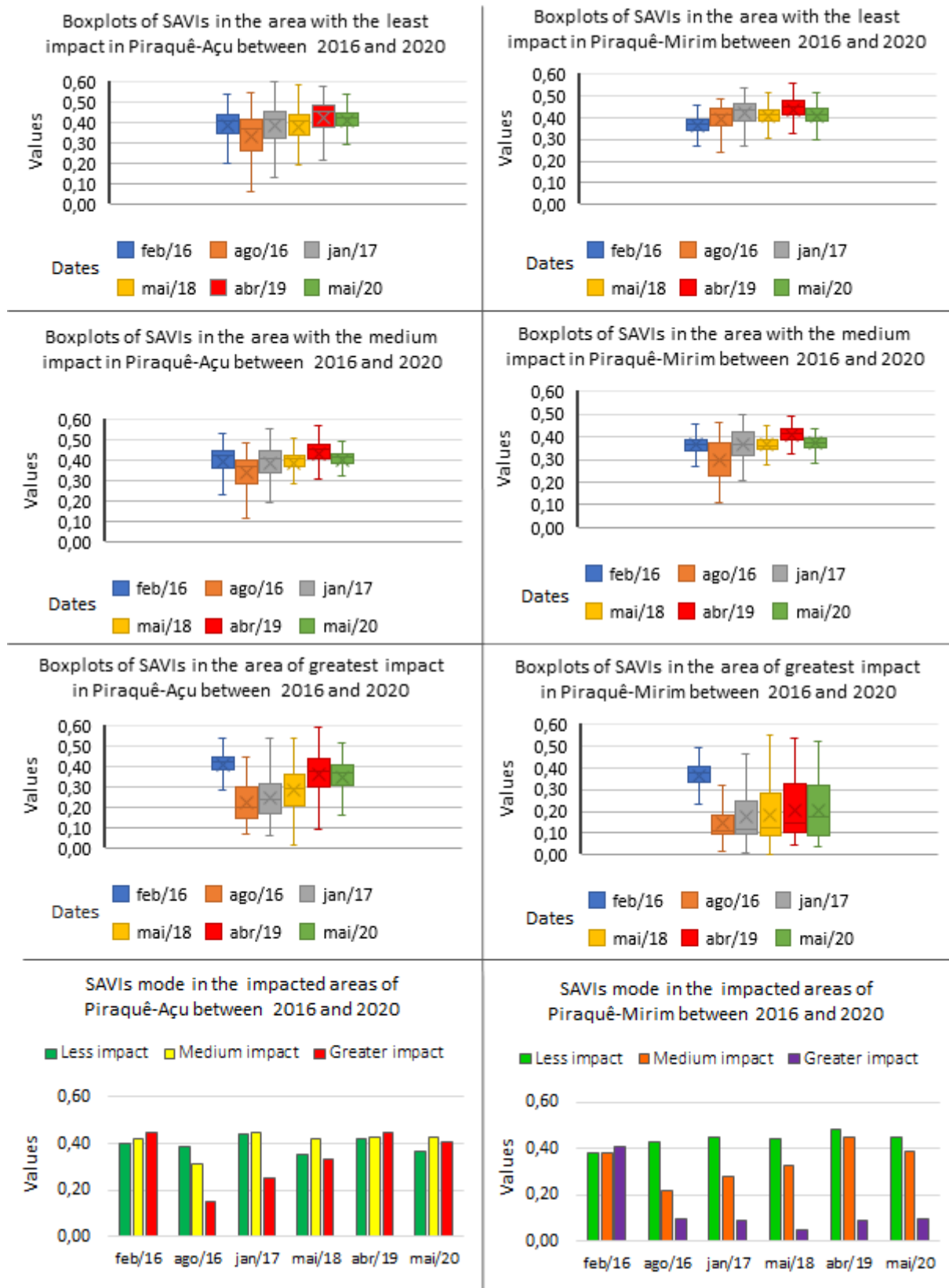
Figure 09 – Graphs with SAVI statistics for the Reserva de Desenvolvimento Sustentável Piraquê Açú-Mirim.
