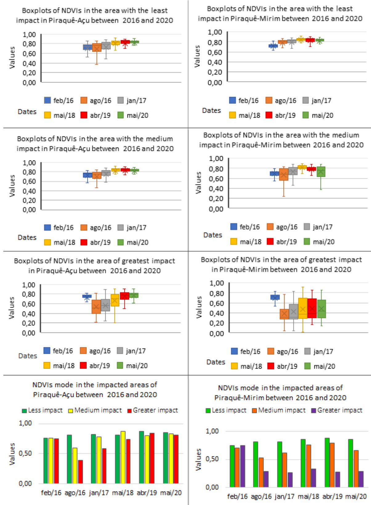
Figure 07 – Graphs with NDVI statistics for the Reserva de Desenvolvimento Sustentável Piraquê Açú-Mirim
