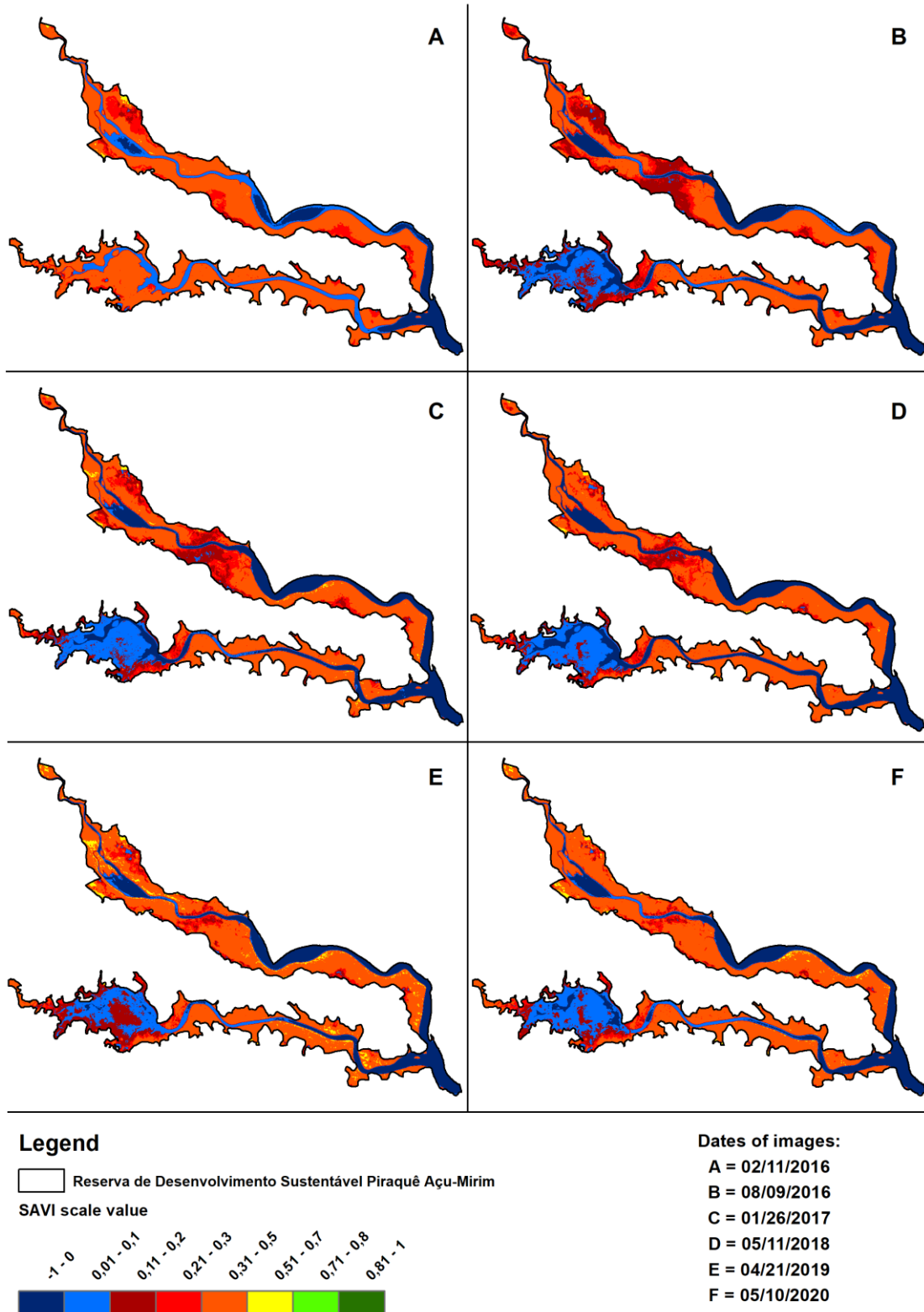
Figure 05 – SAVI of the Reserva de Desenvolvimento Sustentável Piraquê Açú-Mirim, for the years 2016 to 2020.
