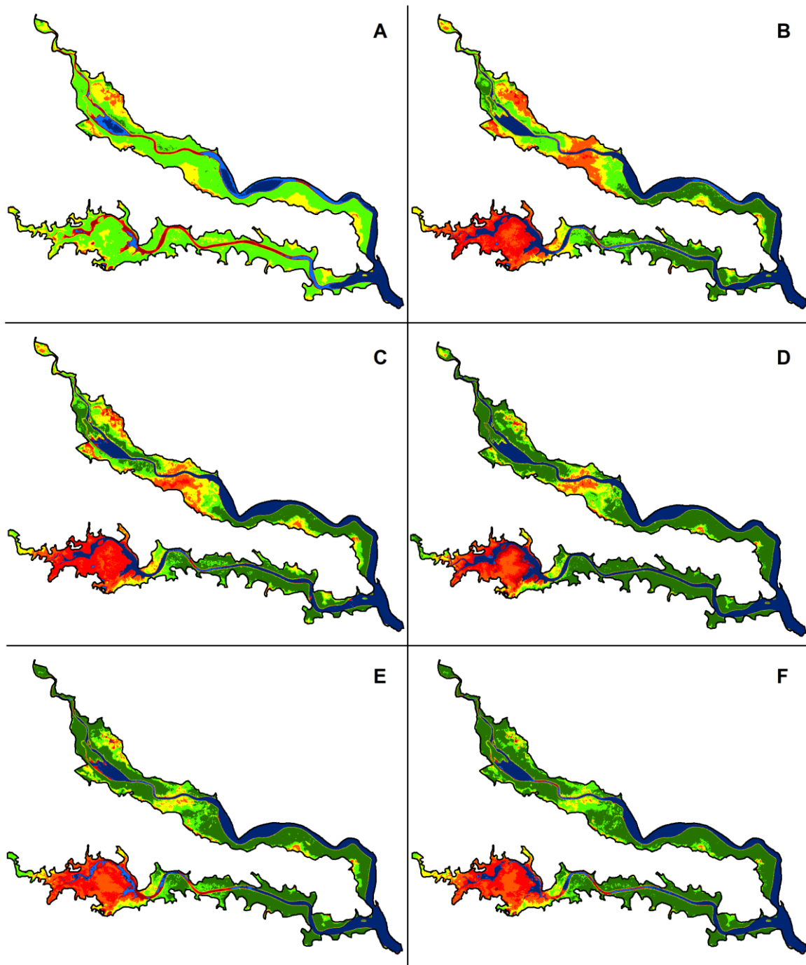
Figure 04 - NDVI of the Reserva de Desenvolvimento Sustentável Piraquê Açú-Mirim for the years 2016 to 2020.
