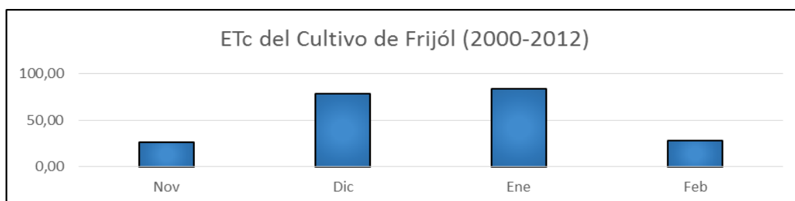
GRÁFICO 3.3 Evapotranspiración real del cultivo del Frijol (mm/mes).
