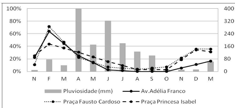
Figura 4. Intensidade da floração de Clitoria fairchildiana Howard em áreas urbanas de Aracaju de novembro de 2009 a março de 2011
