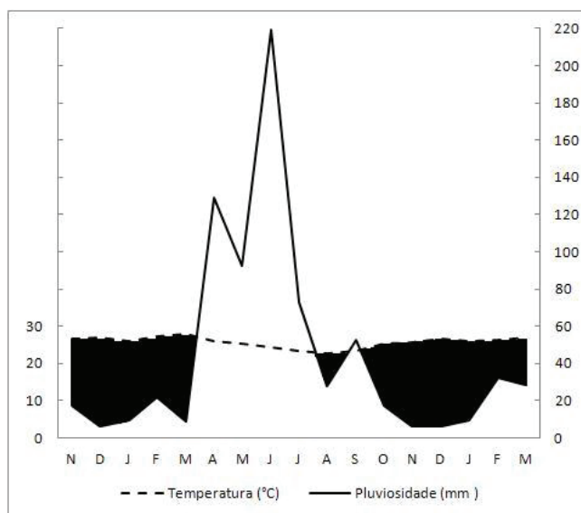
Figura 2. Diagrama ombrotérmico do período de estudo (Novembro de 2009 a Março de 2011) da plataforma de coleta de dados agrometeorológica da cidade de Japarutuba (Longitude: -36.94°, Latitude: -10.59°, 54 m de altitude).
