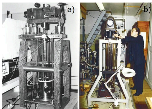
Figura 5 – a) Primeiro protótipo transportável IMGC-BIPM e b) Sakuma operando o equipamento GA-60 em 10 de maio de 1985.
