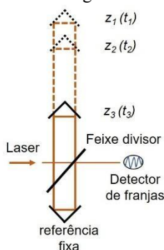
Figura 4 – Princípio de funcionamento de um gravímetro que utiliza a interferometria a laser.
