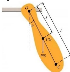
Figura 1 – Pêndulo físico.
