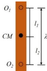
Figura 2 – Pêndulo reversível.
