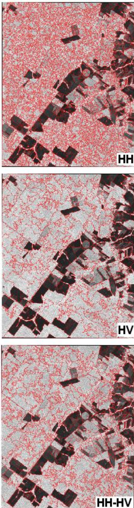
Figura 2 - Segmentação realizada nas imagens HH, HV e HH-HV.
