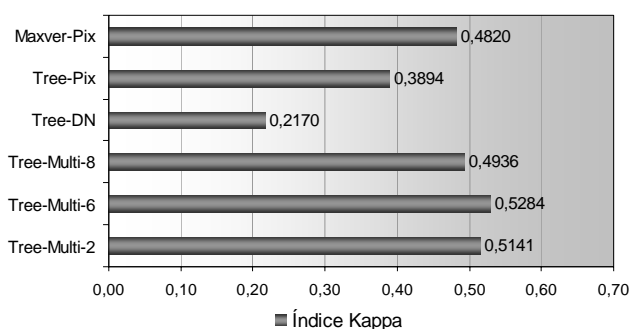
Fig. 14 - Índices Kappa das classificações.
