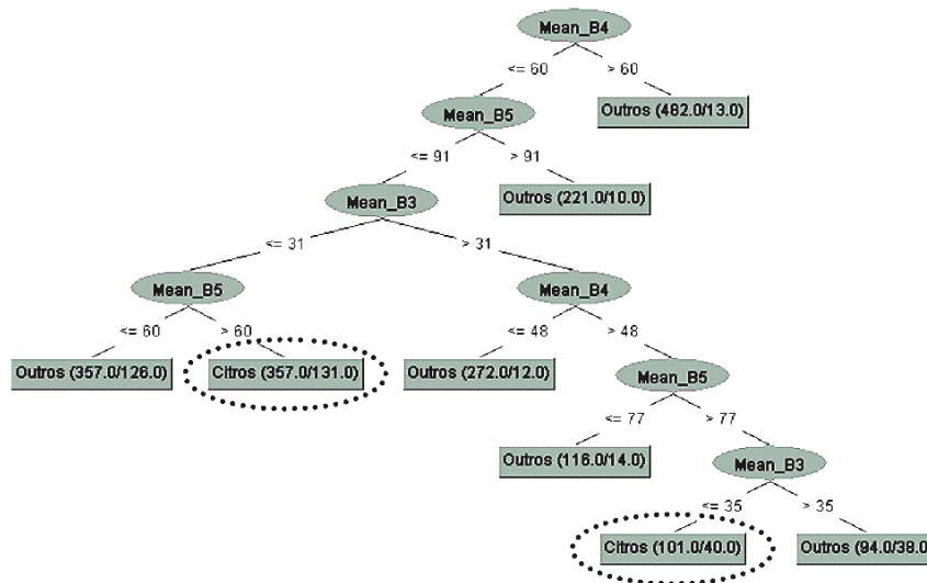
Fig. 9 - Esquema da AD Tree-Pix.
