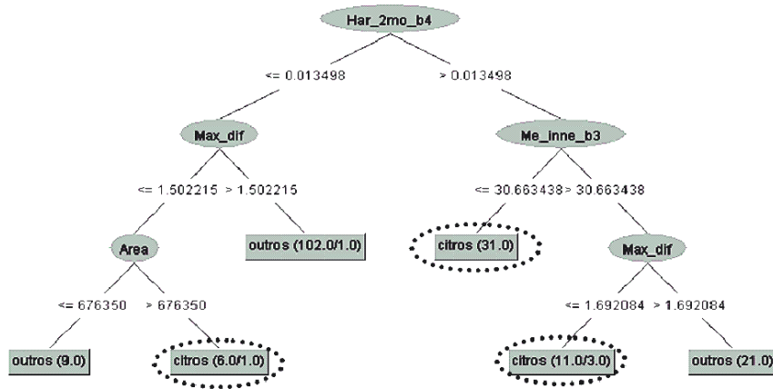
Fig. 6 - Esquema da AD Tree-multi-6.
