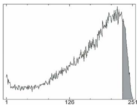
Fig. 10 - Limiarização do histograma do Mapa de Regras por Maxver. Em cinza está a parte aproveitada para a classificação.
