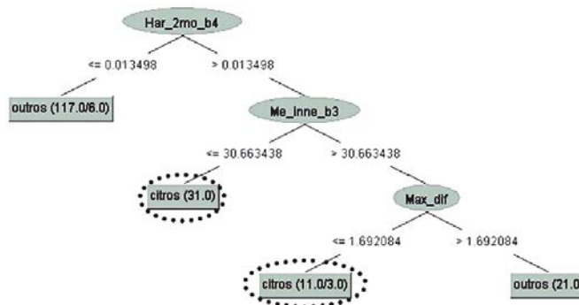
Fig. 7 - Esquema da AD Tree-multi-8.
