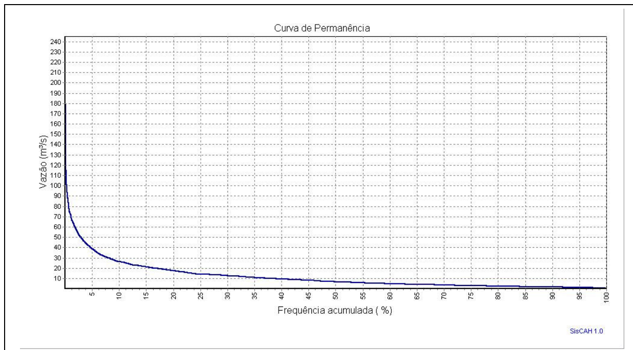
Figura 4. Hidrograma de vazões diárias, totais mensais de pluviosidade e curva de permanência na sub-bacia do rio Uberabinha. (Dados: Agência Nacional de Águas – ANA)
