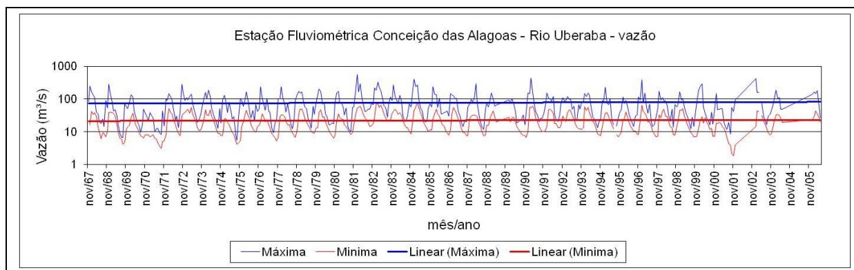
Figura 3. Hidrogramas de vazões diárias, totais mensais de pluviosidade e curvas das permanências na sub-bacia do rio Uberaba. (Dados: Agência Nacional de Águas – ANA)
