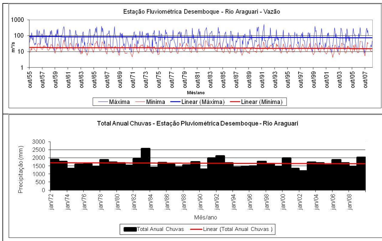
Figura 1. Hidrograma de vazões diárias, totais mensais de pluviosidade e curva de permanência na sub-bacia do rio Araguari. (Dados: Agência Nacional de Águas – ANA)
