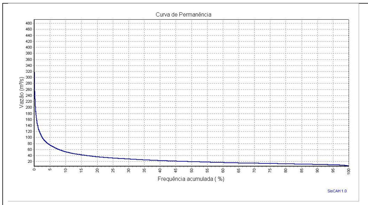
Figura 2. Hidrogramas de vazões diárias, totais mensais de pluviosidade e curvas das permanências na sub-bacia do rio Bagagem. (Dados: Agência Nacional de Águas – ANA)
