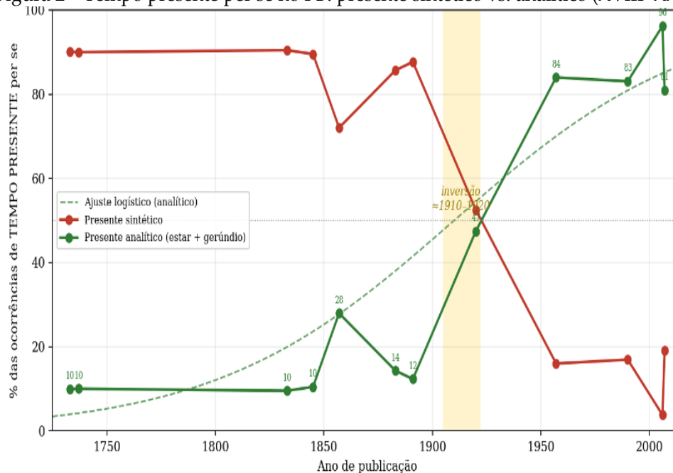
Figura 2 – Tempo presente per se no PB: presente sintético vs. analítico (XVIII–XXI).
