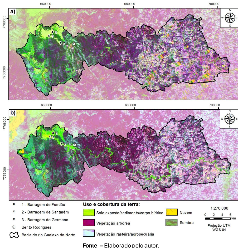
Figura 4 – Imagens resultantes da aplicação da técnica ACP: a) Composição colorida falsa cor RGB CP1 CP2 CP3 para outubro de 2015; b) Composição colorida falsa cor RGB CP1 CP2 CP3 para novembro de 2015.
