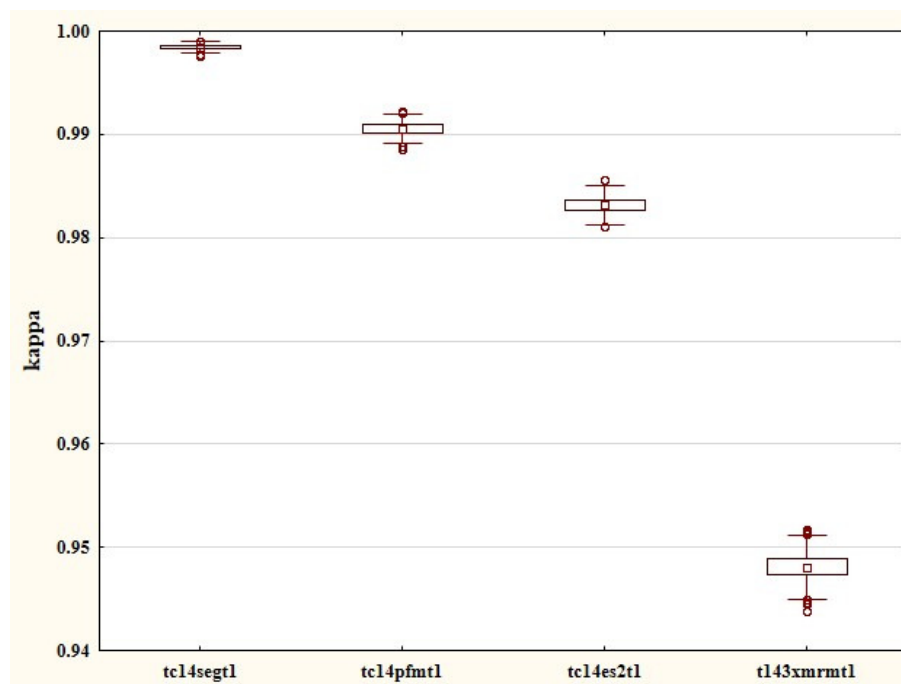
Figura 6: Gráfico de caixa dos valores do coeficiente kappa por procedimento de generalização: Segmentação (tc14segt1), Filtro Moda (tc14pfmt1), Metodologia ESRI (tc14es2t1) e Reamostragem (t143xmrrmt1).
