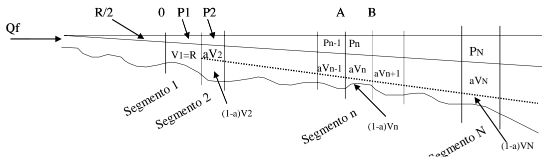
Figura 3 - Modelo hipotético da metodologia de DYER e TAYLOR (1973). P_n e V_n denotam os volumes do prisma de maré e de maré baixa de um segmento genérico n ( a é o parâmetro de mistura), (1-a)V_n é o volume na maré baixa disponível para mistura na maré alta, R é o volume de água fluvial descarregado no estuário durante um período de maré ( T = 43082 segundos para maré semi-diurna), A e B são segmentos hipotéticos.
