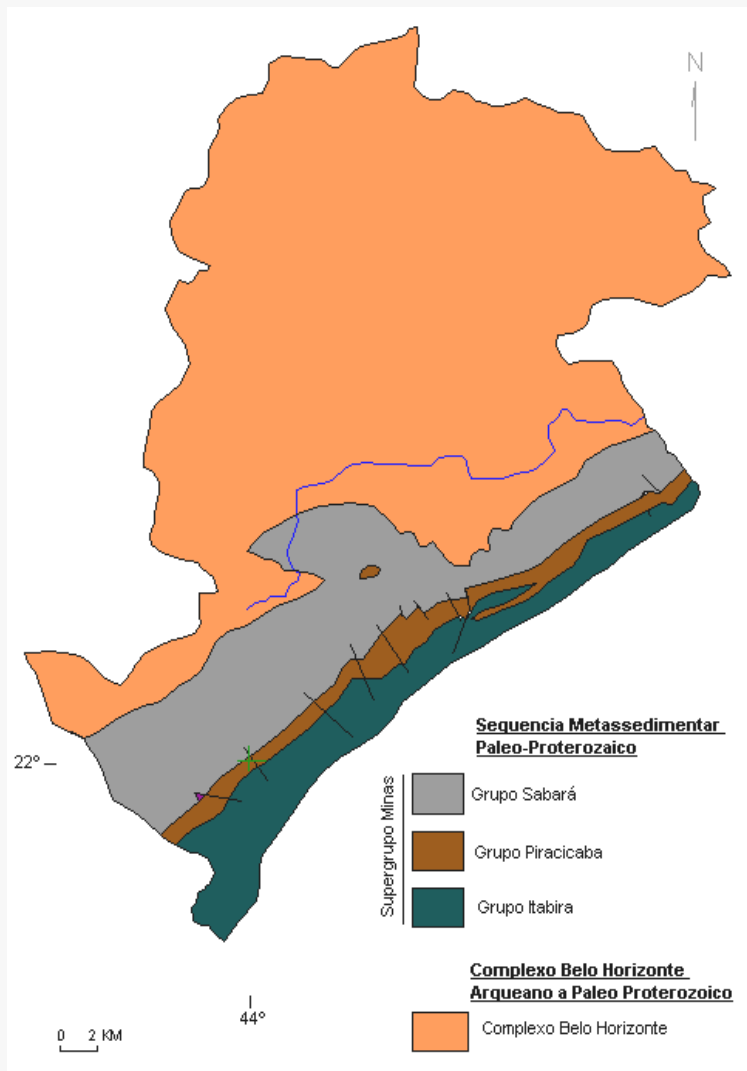
Figura 2 - Mapa Geológico – Geomorfológico de Belo Horizonte
