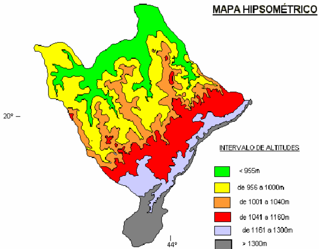
Figura 4 - Mapa hipsométrico da Regional Barreiro, BH (MG)
