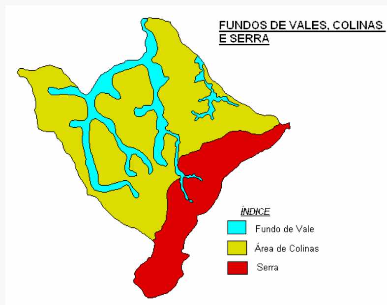
Figura 5 - Mapa dos Fundos de Vales, Colinas e Serras da Reg. Barreiro - BH (MG)
