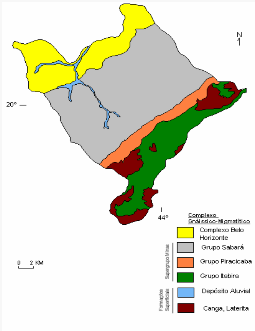
Figura 7 - Mapa geológico da Regional Barreiro
