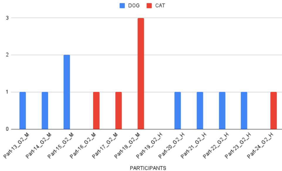
Gráfico 4 – Animais/quantitativo (Grupo 2).
