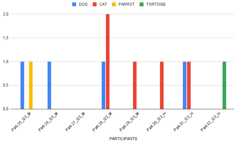
Gráfico 6 – Animais/quantitativo (Grupo 3).
